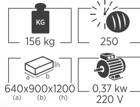
EFE 08-1 YATAY BIÇAKLI OTO. SENSÖRLÜ HORIZONTAL AUTO. BY SENSOR
